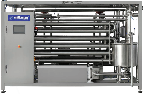
Tubular Pastörizatör / Tubular Pasteurizer Трубчатый пастеризатор / البسترة الأنبوية
